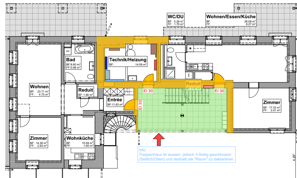
Erdgeschoss
