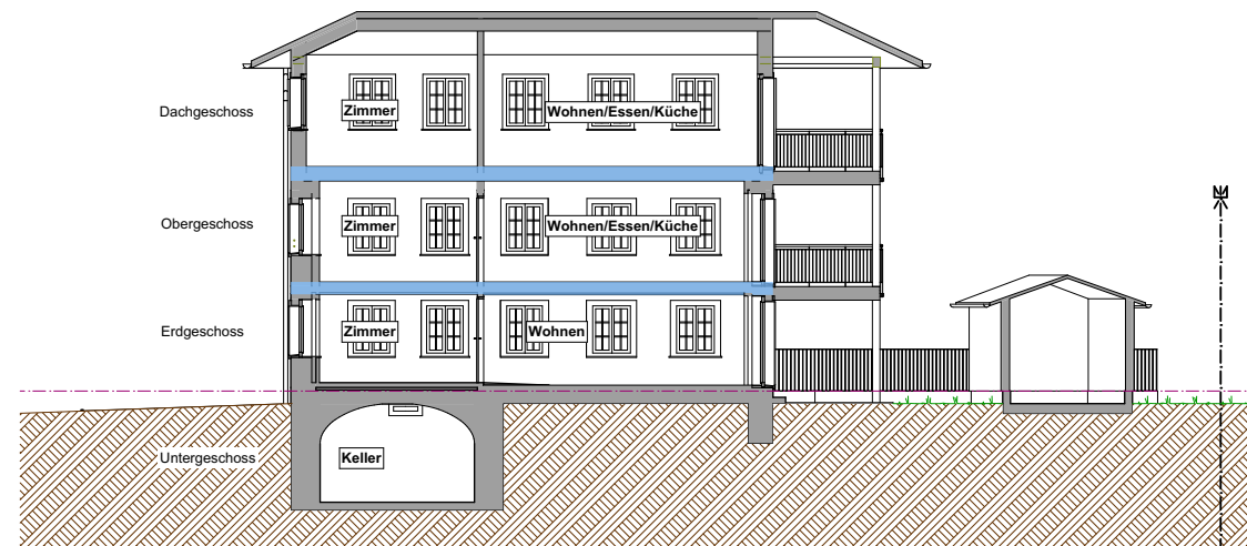
Schnitt A-A
