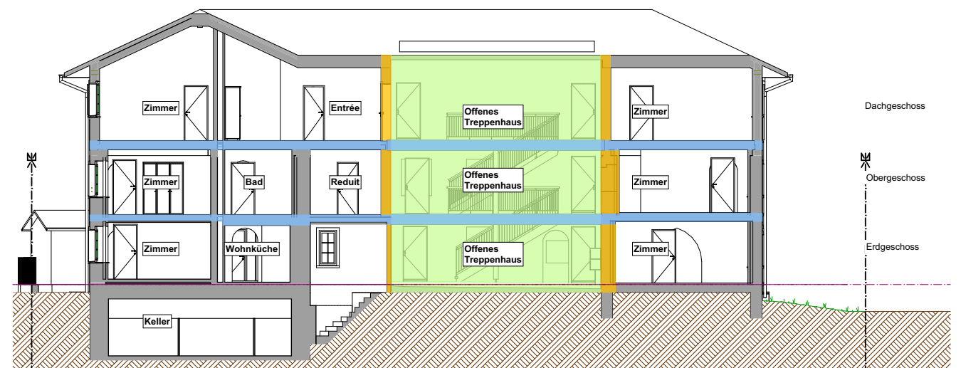
Schnitt G-G
