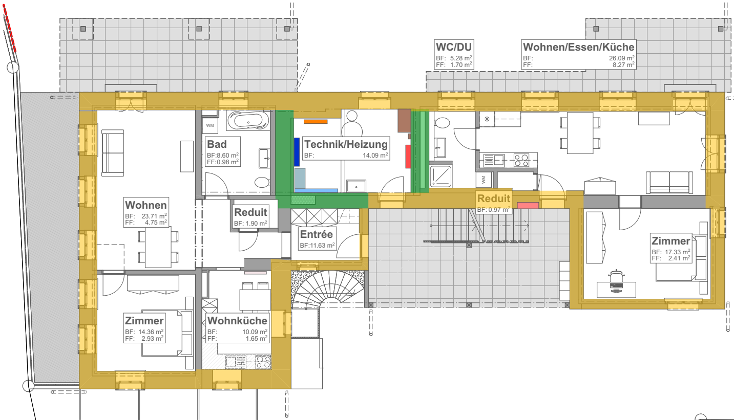
Erdgeschoss
