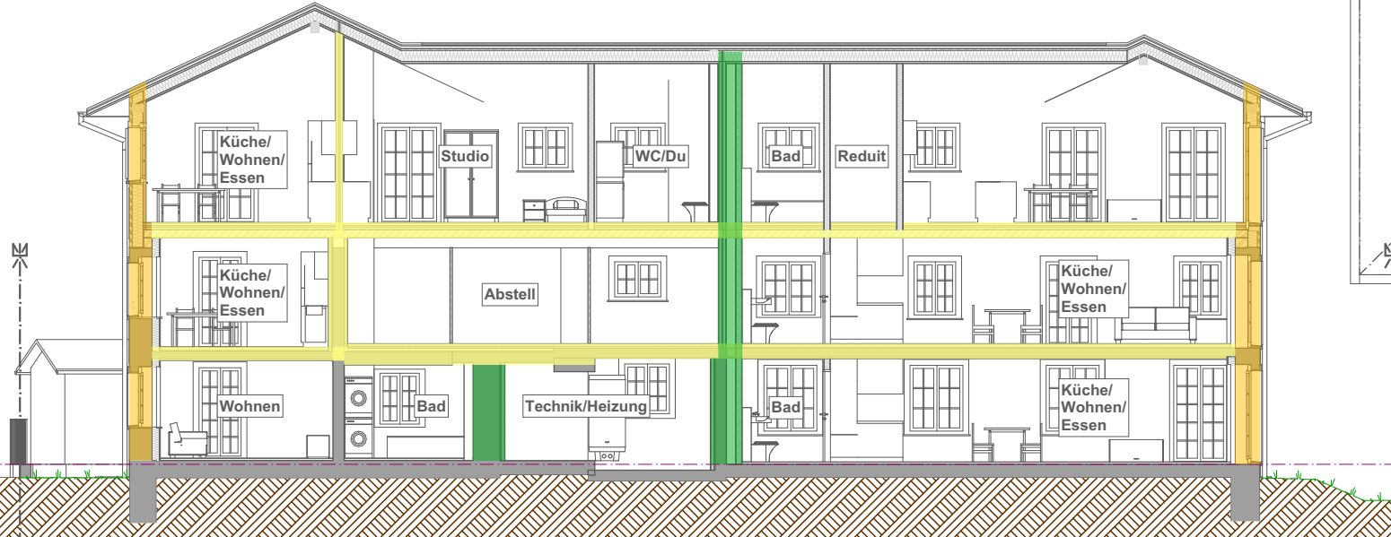
Schnitt E-E
