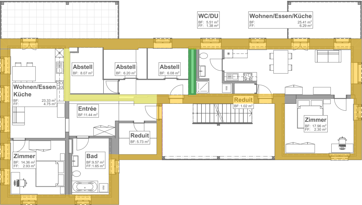
Obergeschoss
