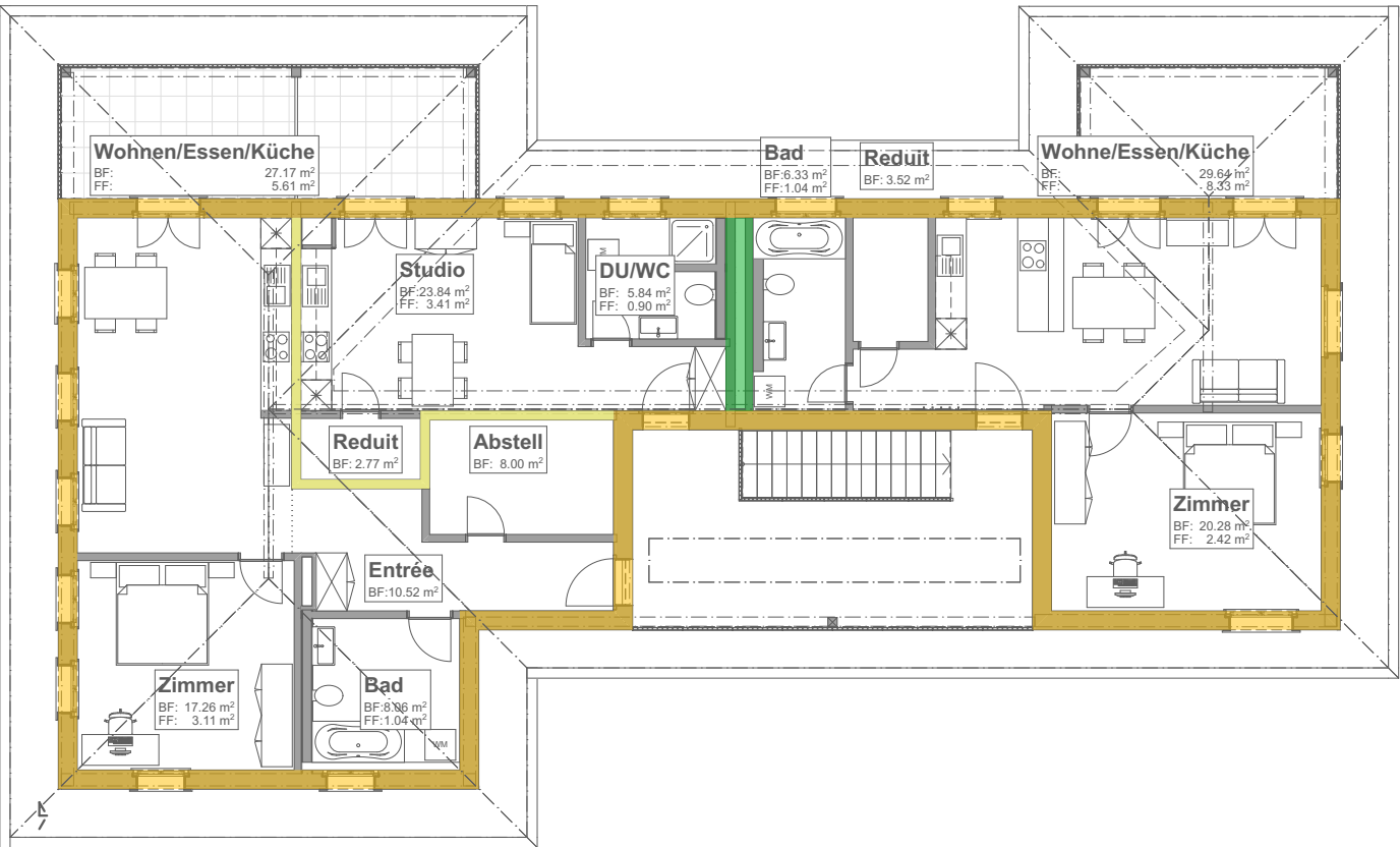
Dachgeschoss
