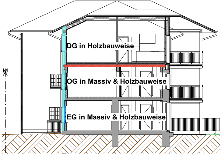
Schnitt D-D
