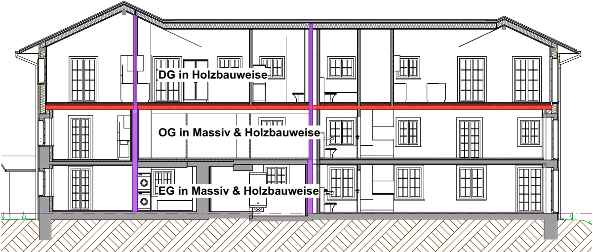
Schnitt E-E
