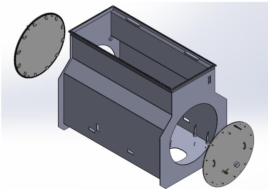
Abbildung 6: Kapselungsdichtigkeits-Prüfsystem HEC 10, CAD-Explosionsdarstellung
