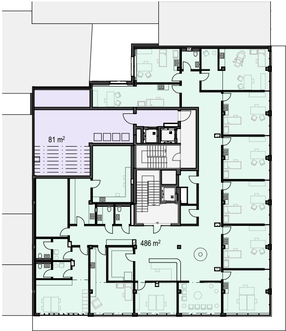
1. Obergeschoss
