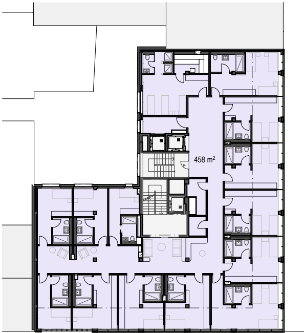
4. Obergeschoss
