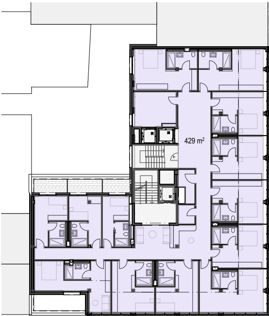
5. Obergeschoss
