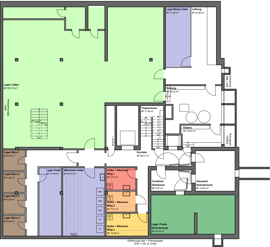
Untergeschoss
