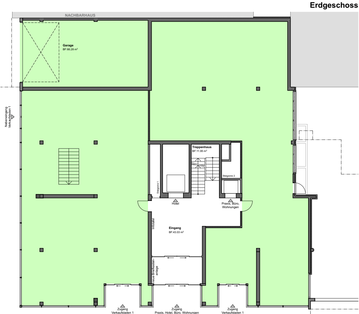
Erdgeschoss
