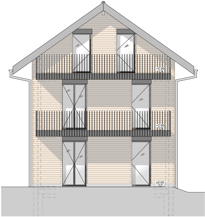
ANSICHT WEST
