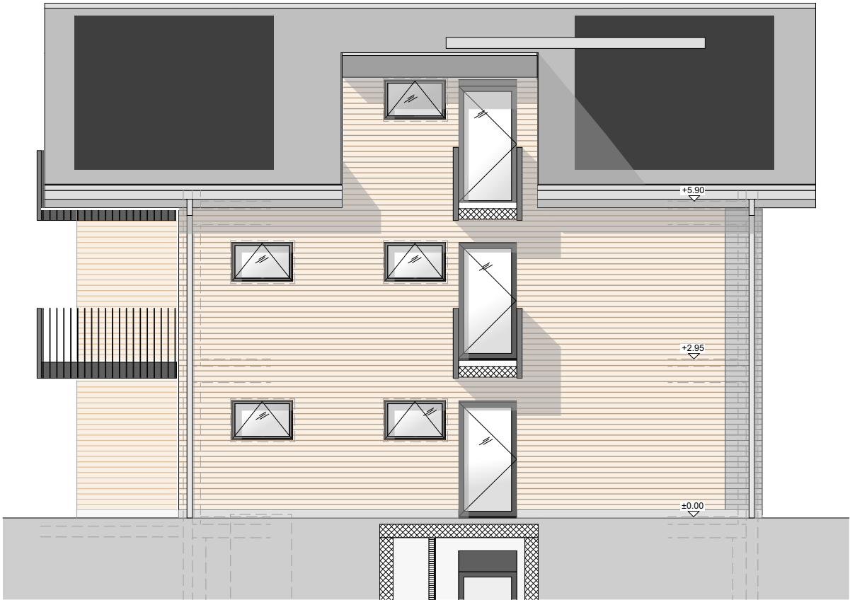
ANSICHT SÜD
