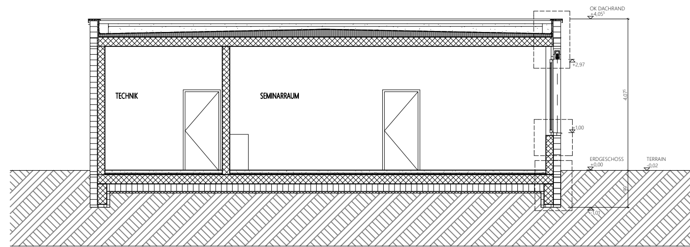
SCHNITT A-A
