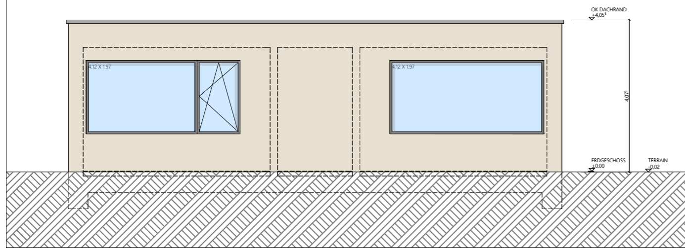
SÜDWESTFASSADE
