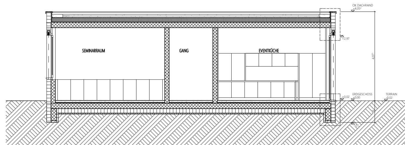
SCHNITT B-B
