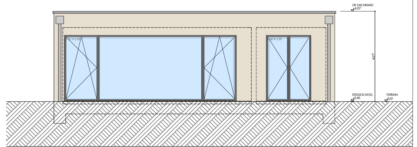
SÜDOSTFASSADE
