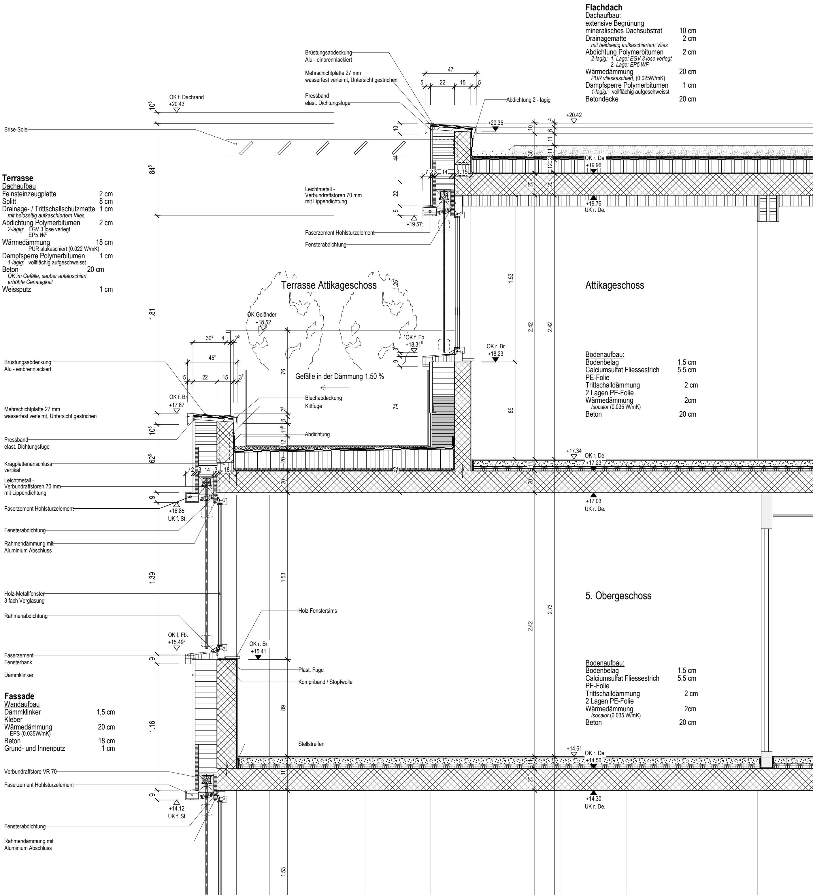
Fassadenschnitt
