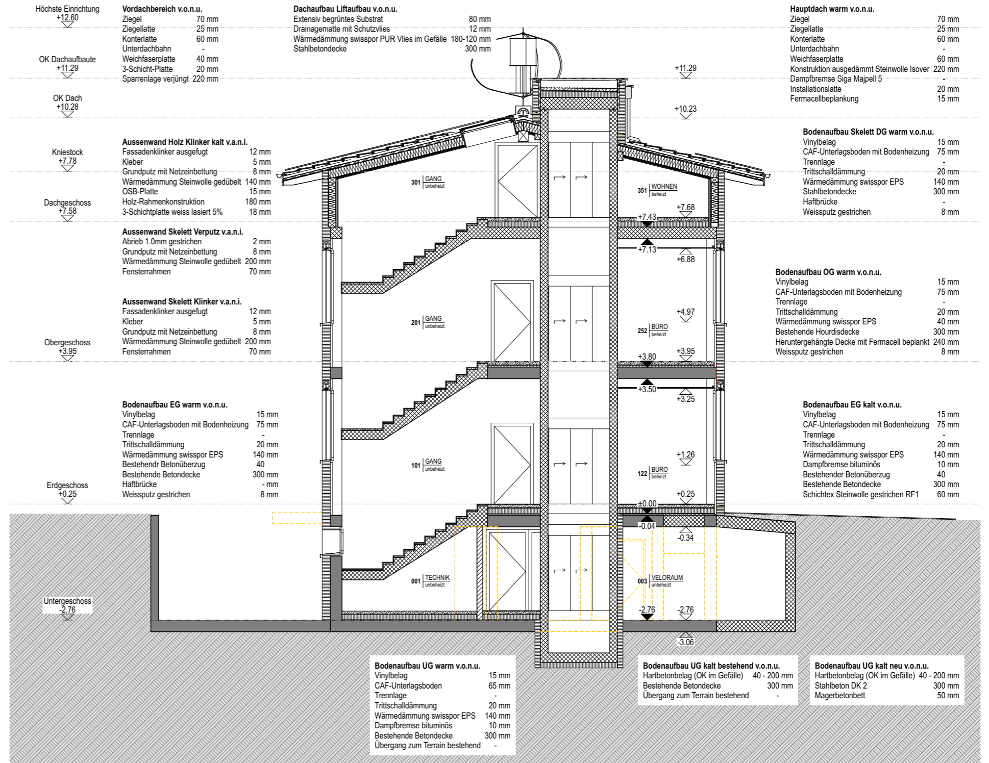
SCHNITT B 1:100
