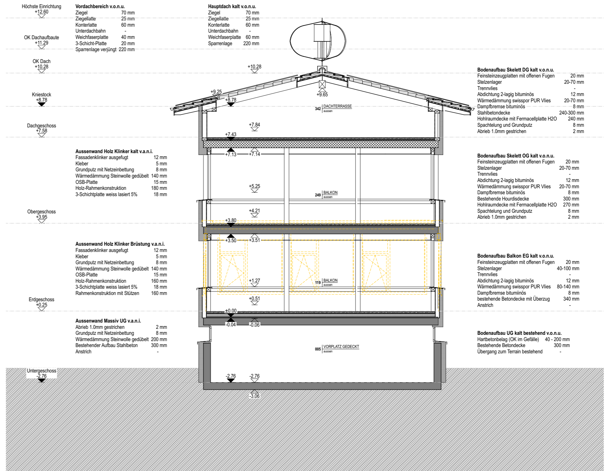
SCHNITT A 1:100
