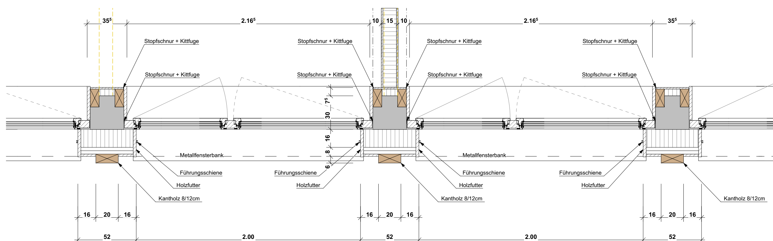
Grundriss Erdgeschoss
