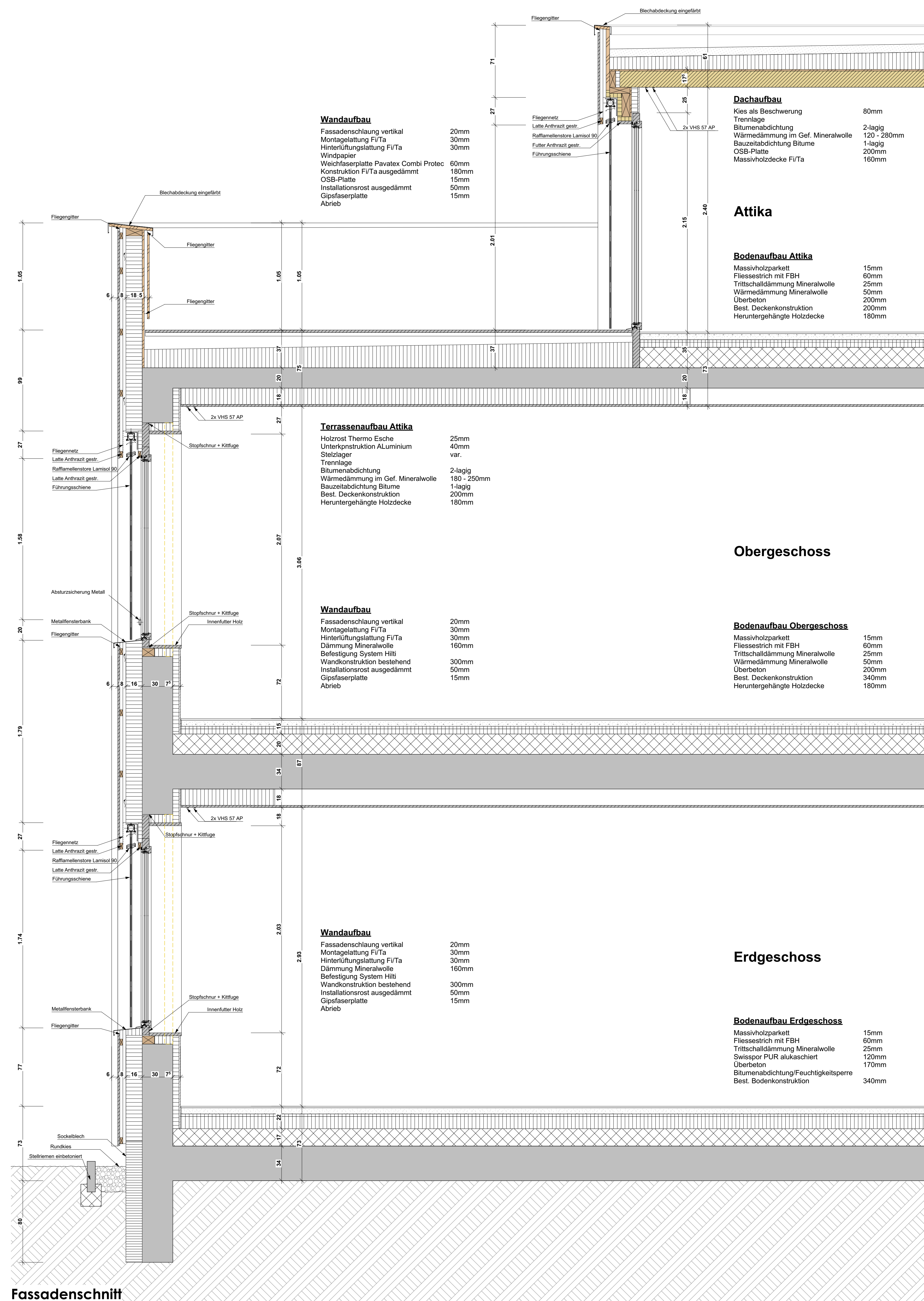
Fassadenschnitt
