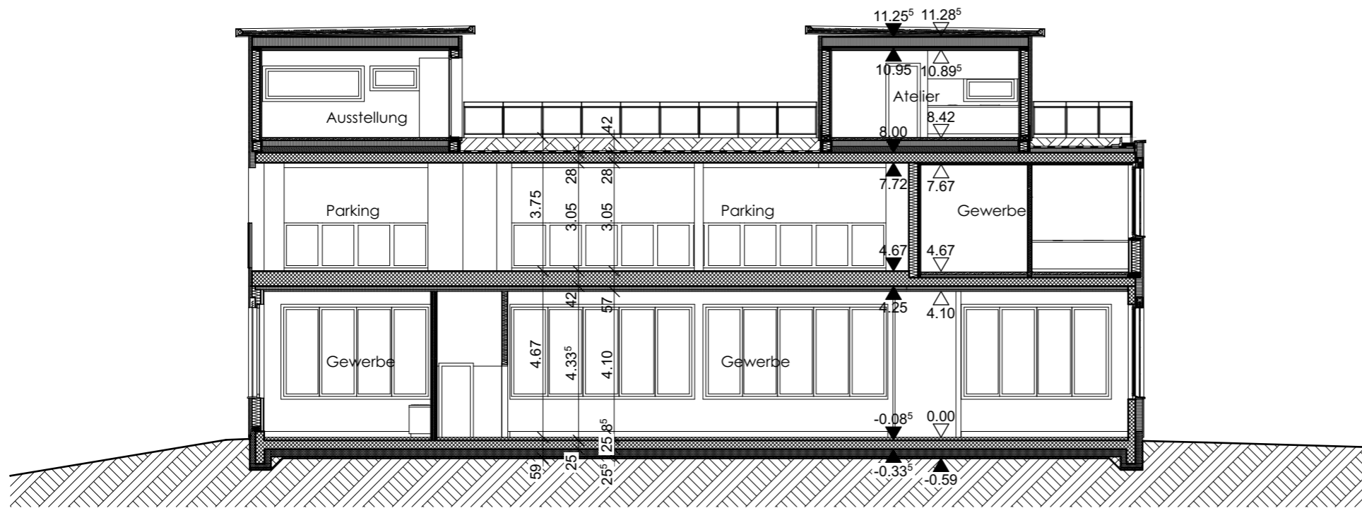
Querschnitt QS1
