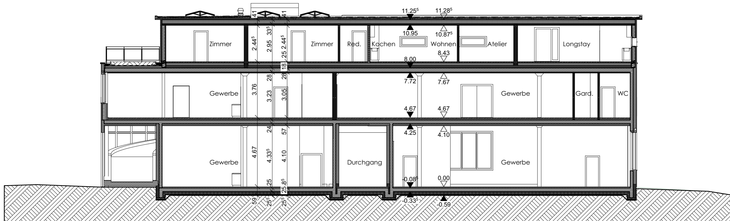
Längsschnitt LS1
